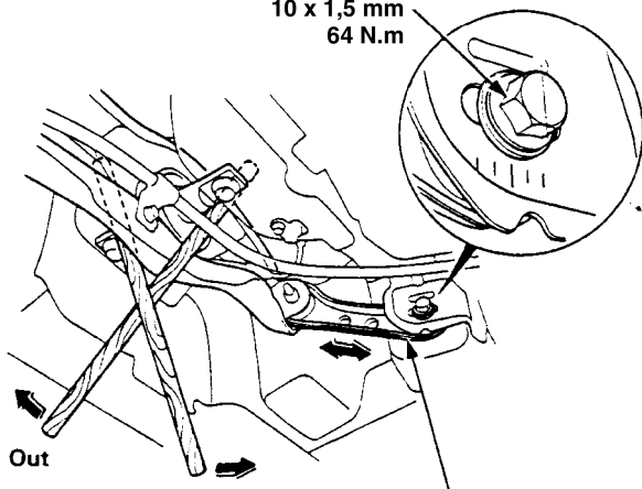
RAMENO KOMPENZÁTORU
